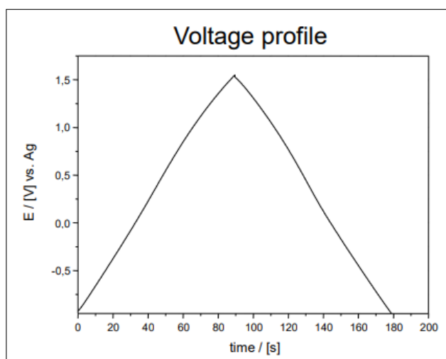
Figura 13: Diagramma carica-scarica
