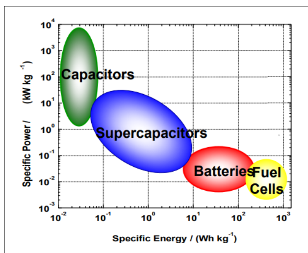
Figura 12: Ragone plot
